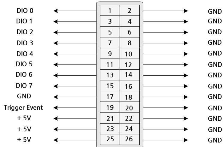
[그림 1-3] COMI-LX203 커넥터 핀 배열
