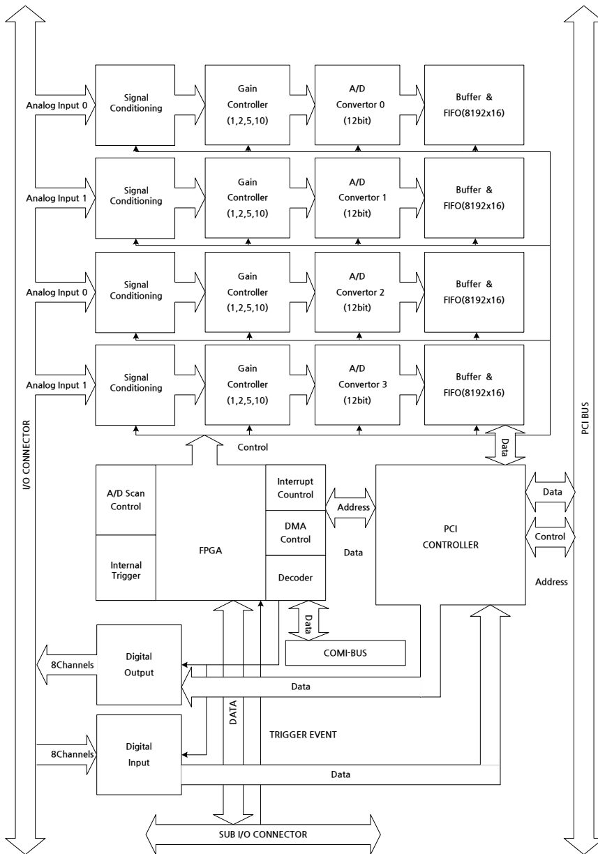
[그림 1-2] COMI-LX203 Hardware 개념도
